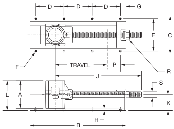
TYPE TUA
