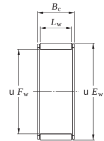
WJ, WJC
