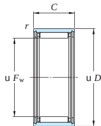
NK ( u F_w \leq 10 )
