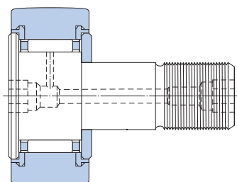
KR .. PPA (22 ≤ D ≤ 26 mm)
